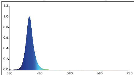
BLEU ((ouverture max.) : Flux=502 lm*
